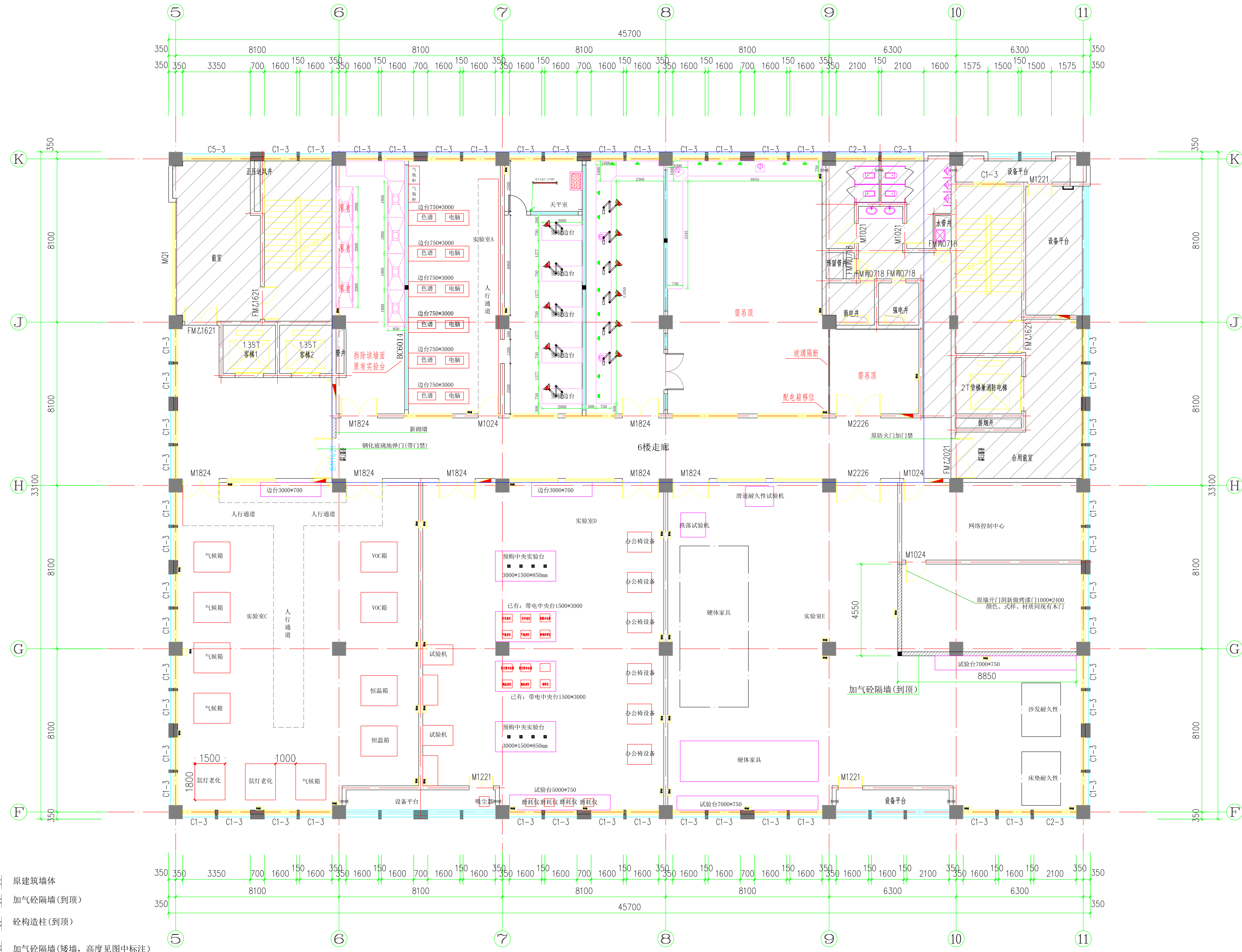
六层平面布置图 1:100
